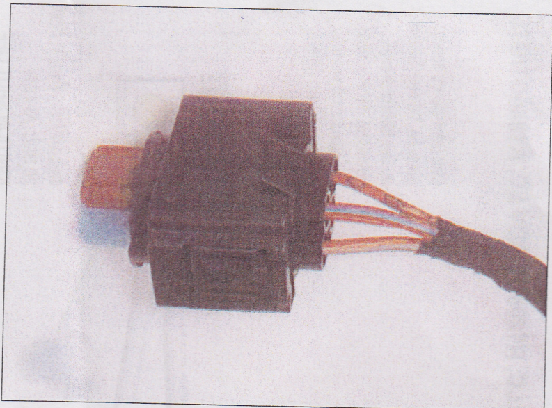
Stecker im Motorrad R1200RT LC / R1200GS LC / R1200GS ADV LC / K1600GT/GTL Exclusive rotes Kabel mit braunem Streifen
